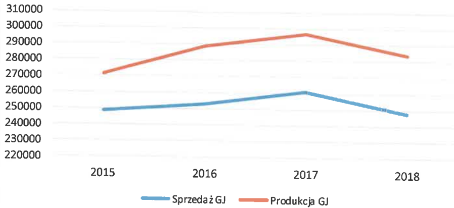
Produkcja i sprzedaż energii cieplnej w latach 2015 - 2018
